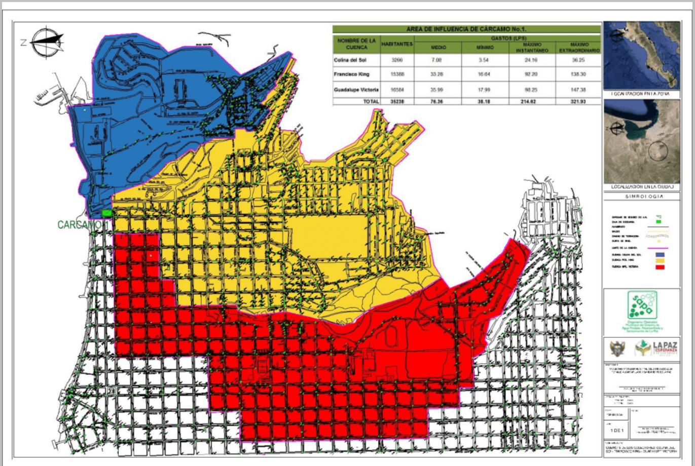
Plano de la red de drenaje y alcantarillado que desembocan en el CÁRCAMO ESTERITO proveniente de las Cuencas COLINA DEL SOL (azul), FRANCICO KING (amarillo) y GUADALUPE (azul) (OOMSAPAS, 2020).
