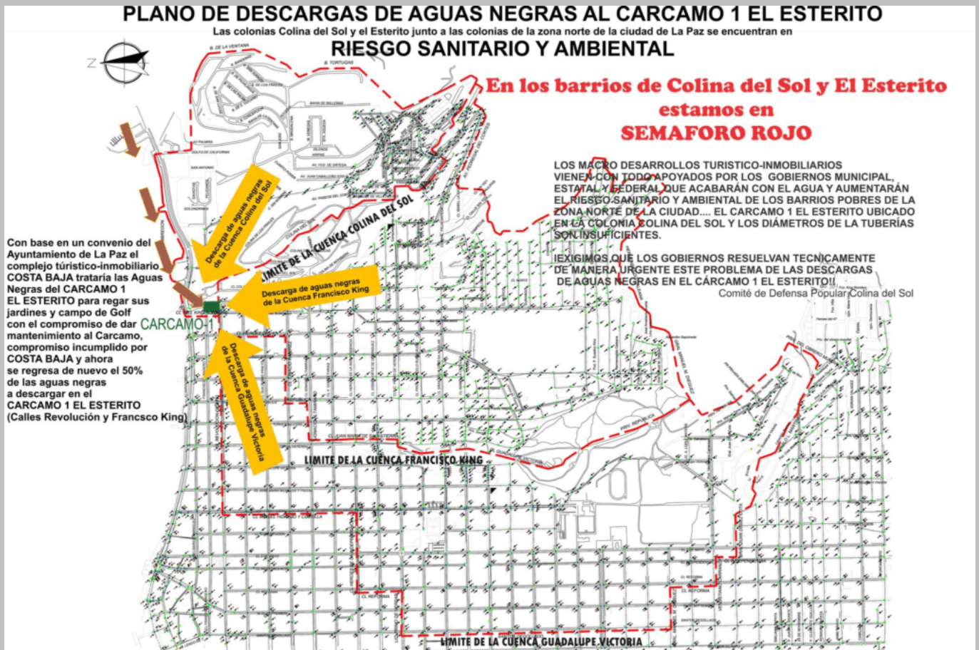
Plano de descarga de aguas negras al CARCAMO ESTERITO que ilustra el riesgo sanitario y ambiental en la colonia Colina del Sol y la bahía de La Paz.(Plano: elaboración propia con base en OOMSAPAS, 2020)
